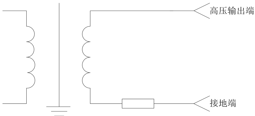
图 1 空载测试示意图
